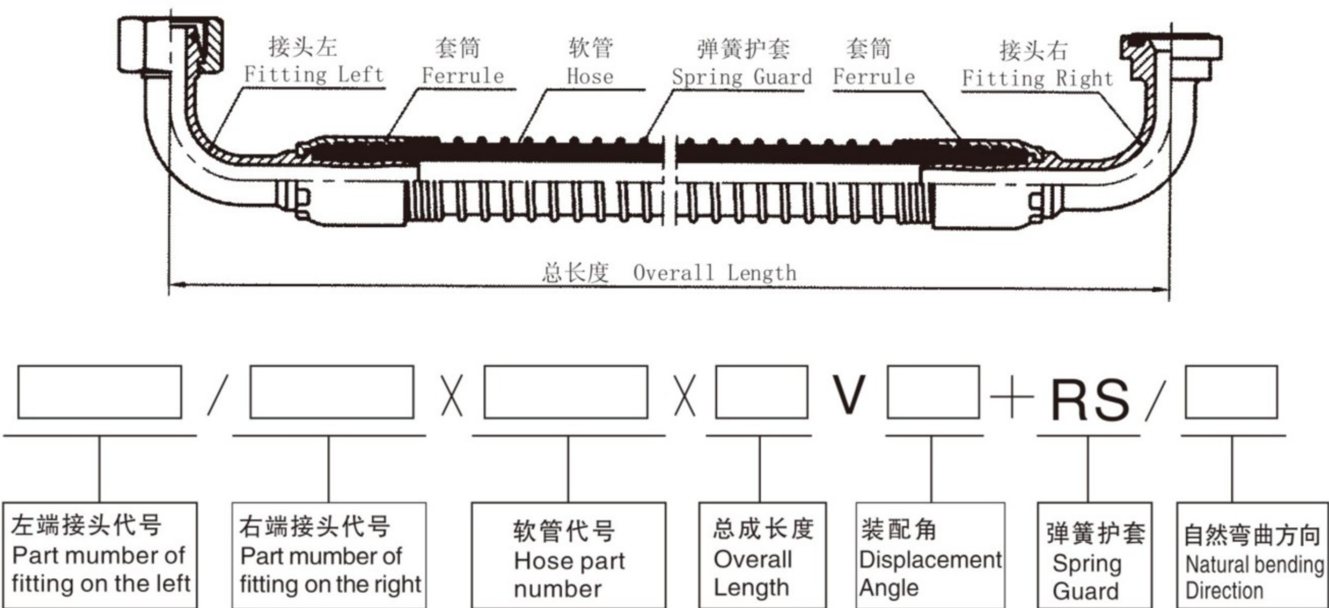
软管总成订货代号
