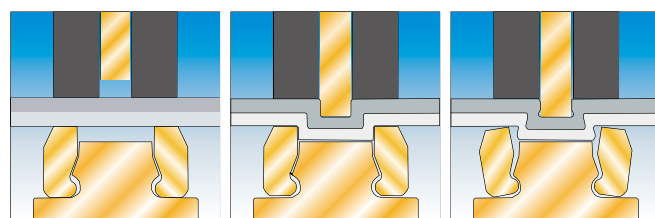
工作原理 Working principle
