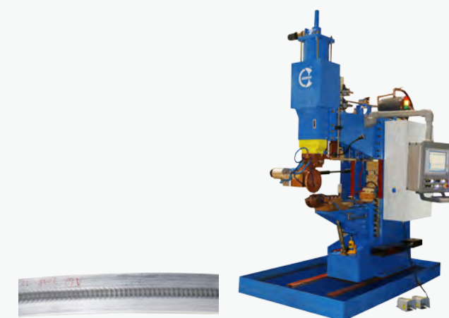
400KVA 中频滚缝焊机 400KVA MFDC Seam Welder
