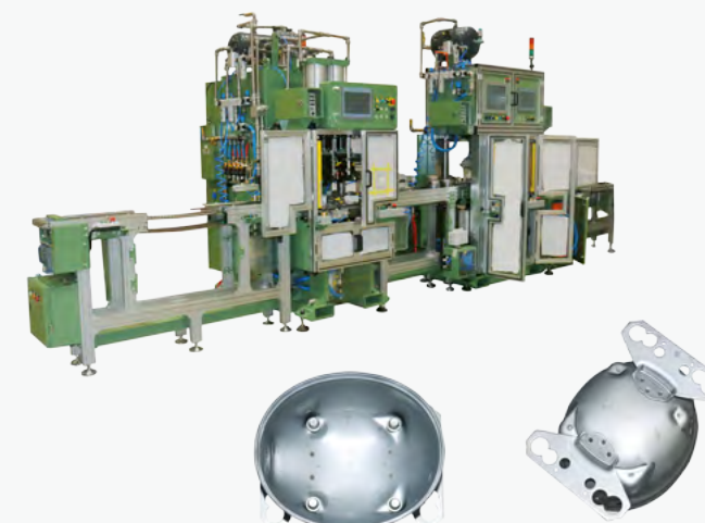
下壳体机脚与销钉自动焊机 Automatic Welder For Base Legs & Pins
