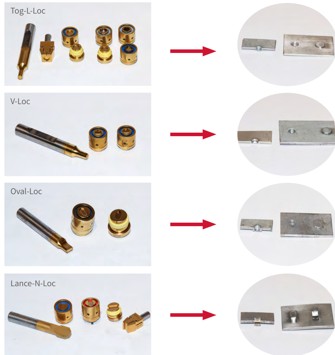
工作原理 Working principle
