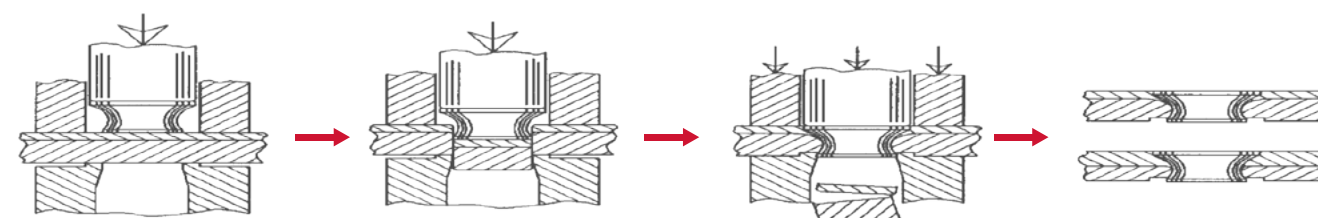
工作原理 Working principle
