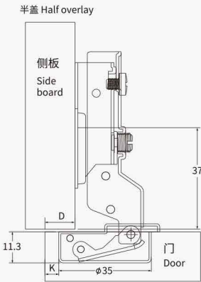
A: 间隙位计算值/gap calculation form
