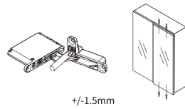
4. 上下方向调节 Up and down adjustment
