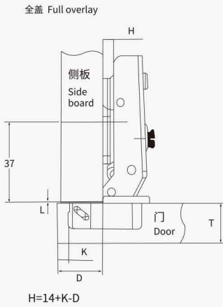
D: 盖位计算值/overlay calculation form
