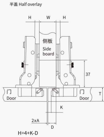
A: 间隙位计算值/gap calculation form
