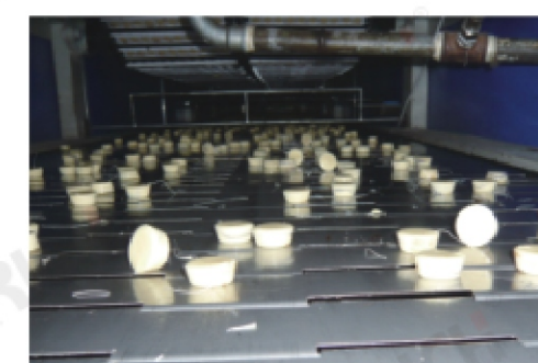
Toffee moulds 太妃糖模具
