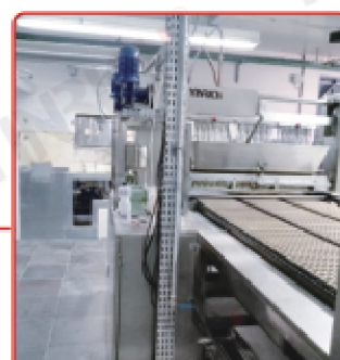
Depositor 浇注机
