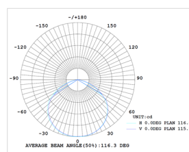
Type III (PC lens)
