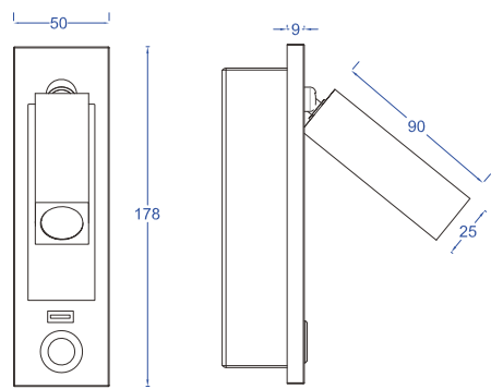
Cutout size : L160 x W40 x H60mm Unit:mm
