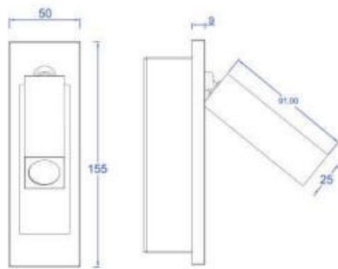
Cutout size : L130 x W40 x H42mm Unit:mm
