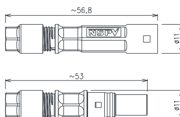
Newsun 1000VDC Mini cable connector:
