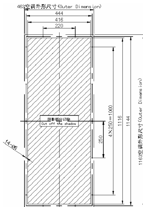
图 5-2 切割示意图 Figure5-2 Cutting diagram
