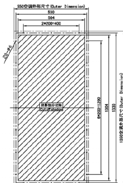
图 5-2 切割示意图 Figure5-2 Cutting diagram
