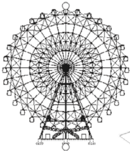
结构简图 | Structure diagram
