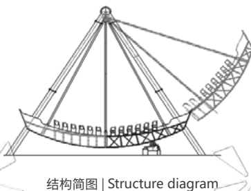
结构简图 | Structure diagram
