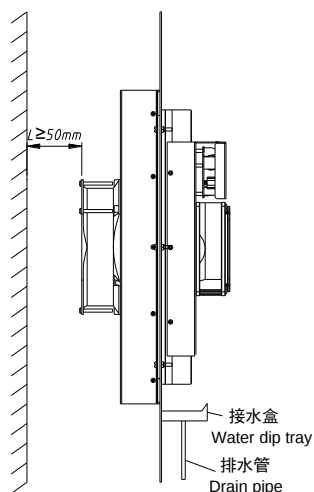
排水示意图
