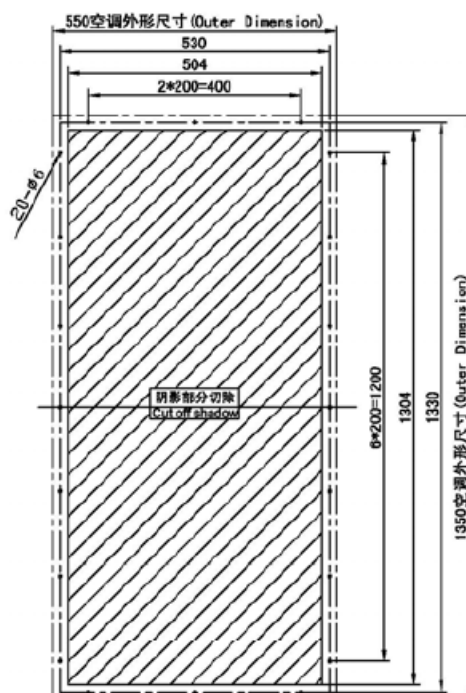
图 5-2 切割示意图 Figure5-2 Cutting diagram
