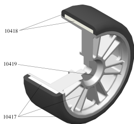
Tyres
