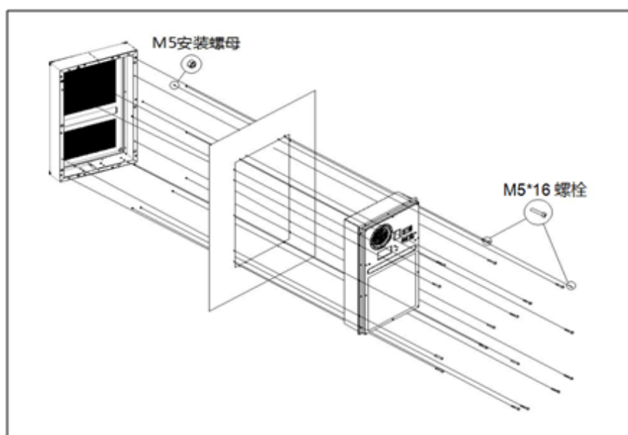
图 5-1 安装示意图 Figure5-1 Installation diagram
