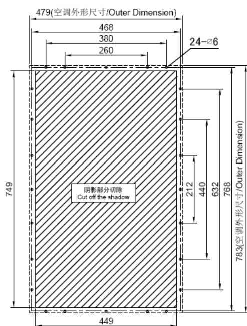
图 5-2 切割示意图 Figure5-2 Cutting diagram
