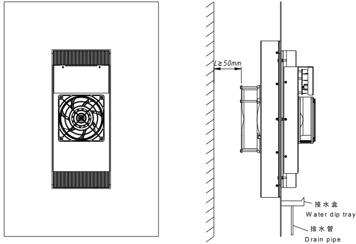
排水示意图 Schematic diagram of drainage
