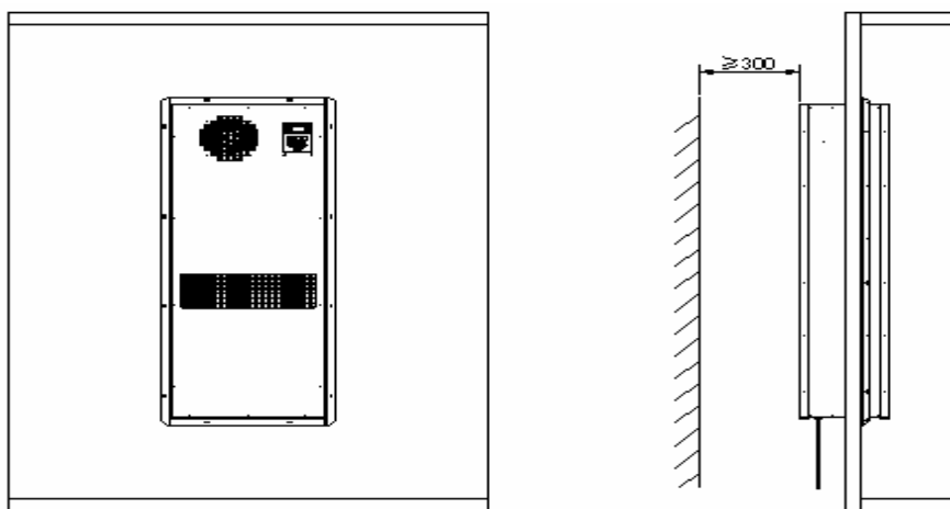
图 5-1 安装示意图 Figure5-1 Installation diagram
