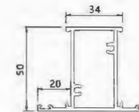
Frame Mullion YLJ35083 T : 2.0mm 1.411kg/m
