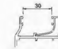
Sash Glass Bead YLJ35104A T : 1.1mm 0.219kg/m
