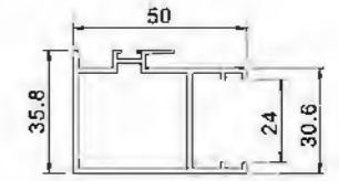
Hook Frame YLJ188C07BZK T=1.4mm 0.71kg/m
