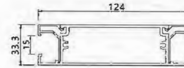
Leaf Cross Bar YLJ37030 T : 2.0mm 1.739kg/m YLJ37029 T=1.2mm 0.23kg/m
