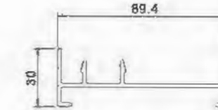
Edge Frame L850720 T=2.0mm 0.990kg/m
