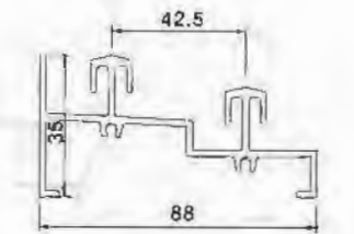
Bottom Rail YLJ388A02B T=2.0mm 1.511kg/m
