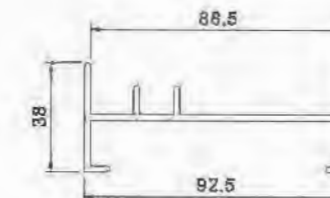
Edge Seal YLJ388A03 T=2.0mm 1.074kg/m
