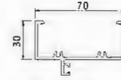
Above YLJ37021 T : 2.0mm 0.943kg/m YLJ37021A T=1.4mm 0.726kg/m
