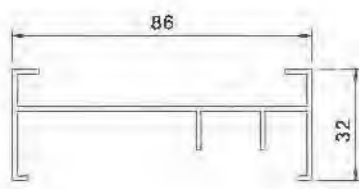
Edge L85A0814 T=1.4mm 0.716kg/m
