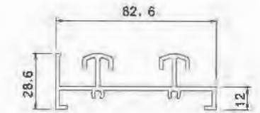
Bottom Groove CG8511F T=2.0mm 1.209kg/m
