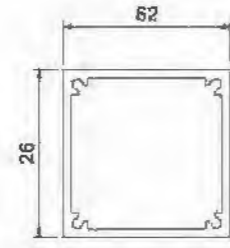
Column YLJ82091 T=3.0mm 2.106kg/m
