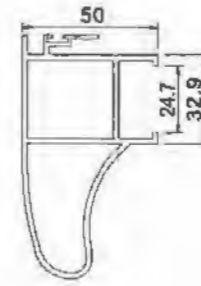
Hook Frame YLJ388A07BZK T=2.0mm 1.67kg/m
