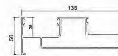
Edge YLJ313503 T=2.0mm 2.083kg/m
