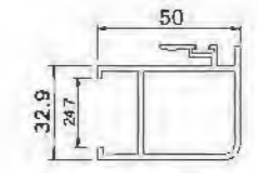
Hook Frame YLJ388A07HZK T=2.0mm 1.036kg/m
