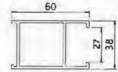
Vertical Frame YLJ37026AZK T : 2.0mm 1.074kg/m
