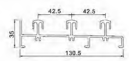
Bottom Rail YLJ388A02G T=2.0mm 2.026kg/m
