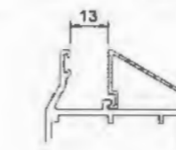
Frame Glass Bead YLJ35085 T : 1.0mm 0.178kg/m
