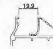
Sash Glass Bead YLJ35085A T : 1.0mm 0.167kg/m
