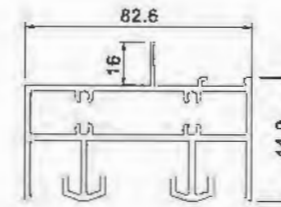
Upper Groove L85A0220 T=2.0mm 2.082kg/m
