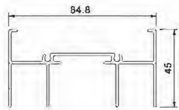
Upper Groove L851414 T=1.4mm 0.991kg/m
