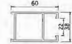
Vertical Frame YLJ37026ZK T : 2.0mm 1.113kg/m
