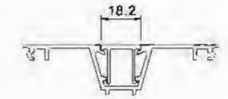
YLJ815C07 T=1.2mm 0.314kg/m
