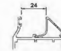
Sash Glass Bead YLJ35104B T : 1.1mm 0.174kg/m
