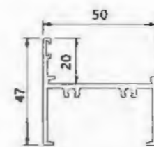
Horizontal Frame YLJ35081 T : 1.9mm 0.785kg/m
