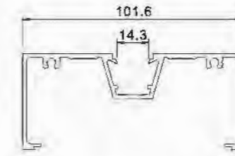
YLJ815C01 T=1.8mm 1.4kg/m
