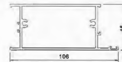
Sash Bottom YLJ35105 T : 2.0mm 1.697kg/m
