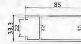
Door Leaf YLJ37015ZK T : 2.0mm 1.424kg/m
