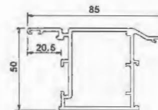
Door Leaf YLJ35083D T : 2.0mm 1.42kg/m
