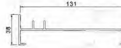
Edge Seal YLJ388A03G T=2.0mm 1.306kg/m
