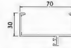
Frame Edge YLJ37023 T : 2.0mm 0.85kg/m YLJ37023A T=1.4mm 0.633kg/m
