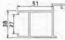
Double Sash Middle Frame YLJ37027AZK T : 2.0mm 1.184kg/m
