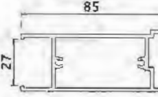
Door Leaf YLJ37015AZK T : 2.0mm 1.385kg/m
