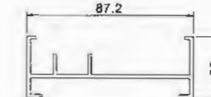
Edge Frame CG8513F T=2.0mm 0.968kg/m
