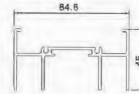
Upper Groove L852020 T=2.0mm 1.369kg/m
