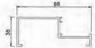
Edge Seal YLJ388A03 T=2.0mm 0.941kg/m
