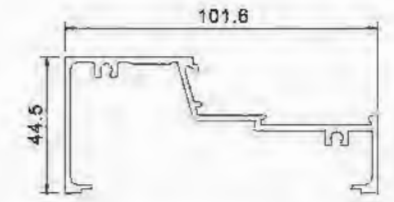
YLJ815C04 T=1.8mm 1.197kg/m
