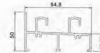
Bottom Groove L851320 T=2.0mm 1.536kg/m
