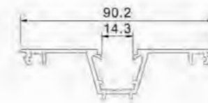
YLJ815C03 T=1.8mm 0.781kg/m
