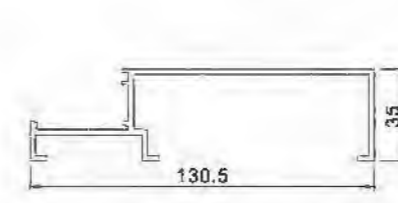
Edge Seal YLJ388A03C T=2.0mm 1.285kg/m
