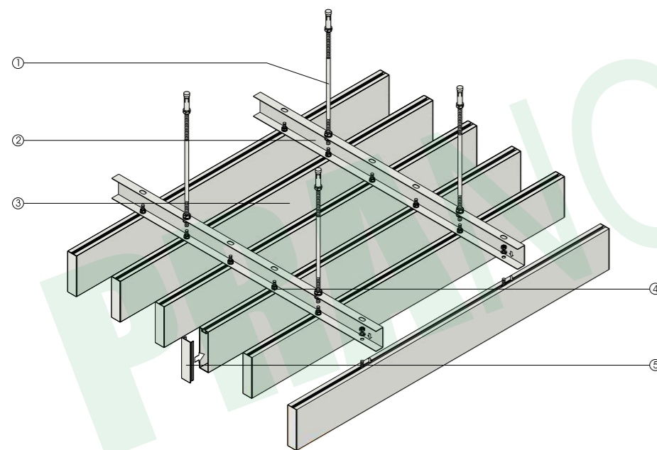
龙骨连接图
