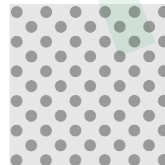
孔径 hole size:3.0mm斜排孔
