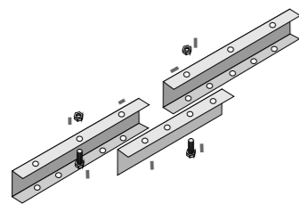
方条型吊式天花吊挂系统示意图
