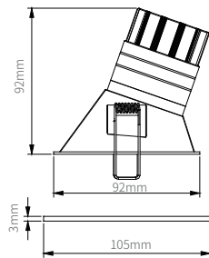
GE-05111-8W-105-H27K90WH
