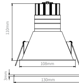
GE-05112-8W-130-H27K90WH
