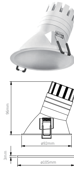
GE-05102-8W-105-H27K90WH
